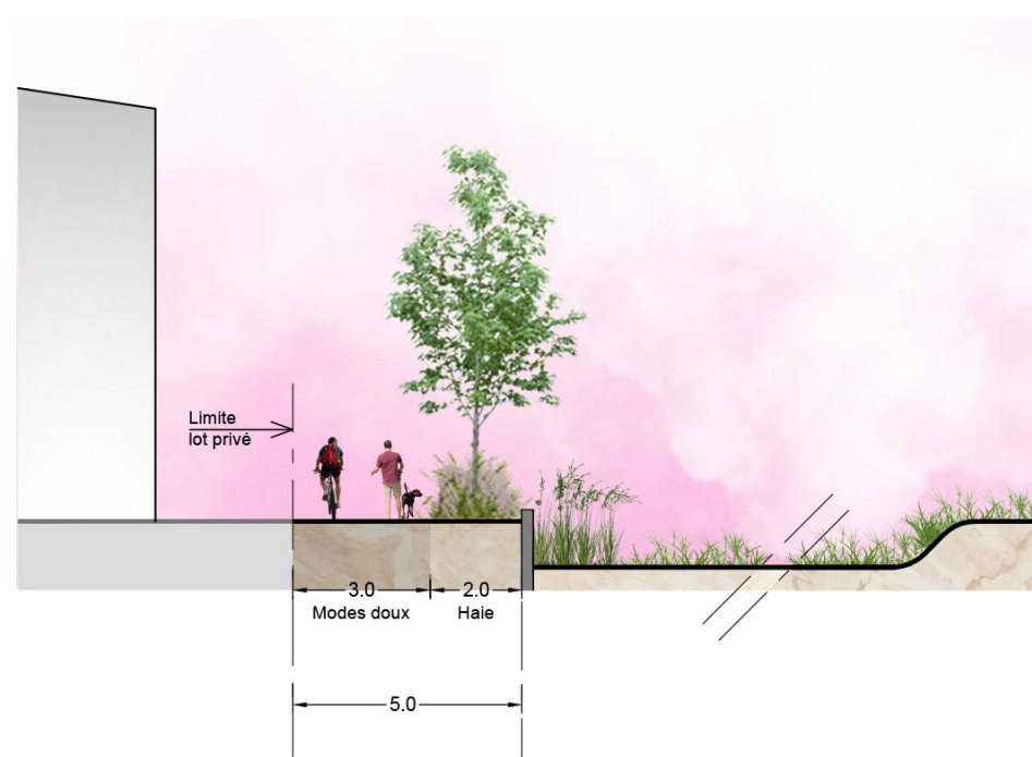
Profil bordant le bassin de rétention
