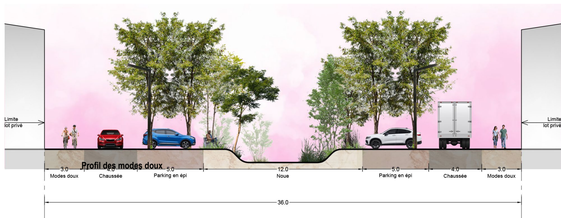
Profil sur noue et mail planté
