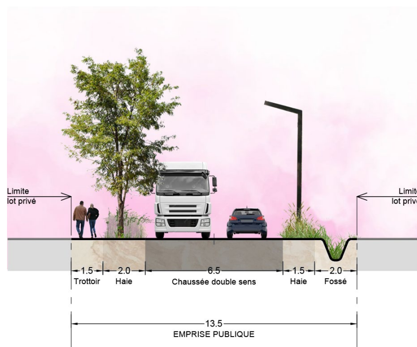
Profil type de desserte
